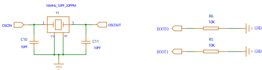
晶振电路
