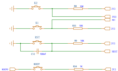
按键电路
