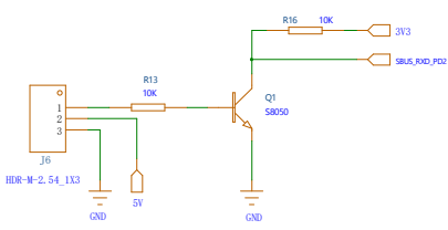
S.BUS航模遥控接口
