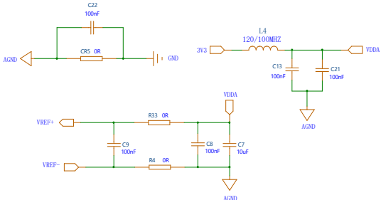
VET6 外围电路
