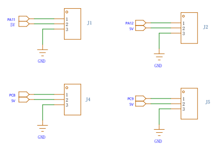
4路舵机
