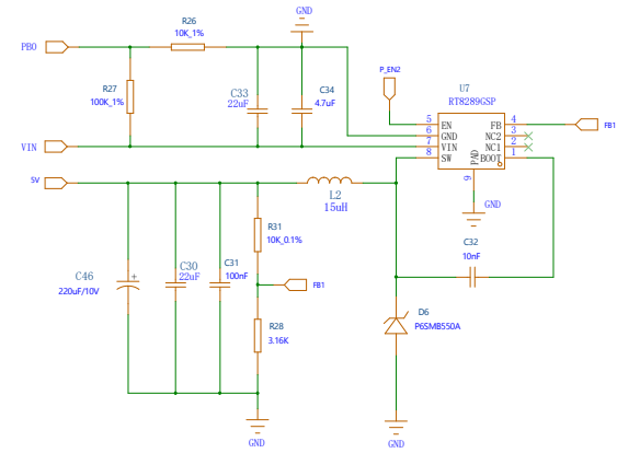
板载5V电源电路
