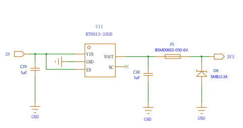
5V 转3.3V 电路
