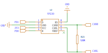
CAN 接口
