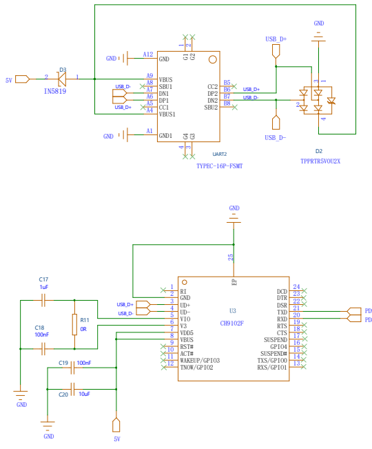
串口3电路
