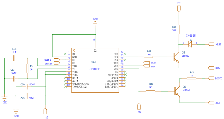
串口1/下载接口电路
