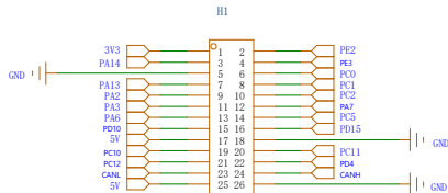
扩展接口
